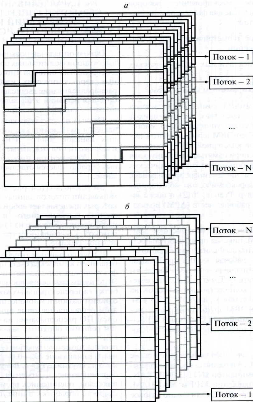
Рис. 2. Иллюстрация основных подходов, используемых для распознавания вычислений при обработке гиперспектральных и многоспектральных изображений: a – параллельная обработка фрагментов; б – параллельная обработка групп спектральных каналов.
