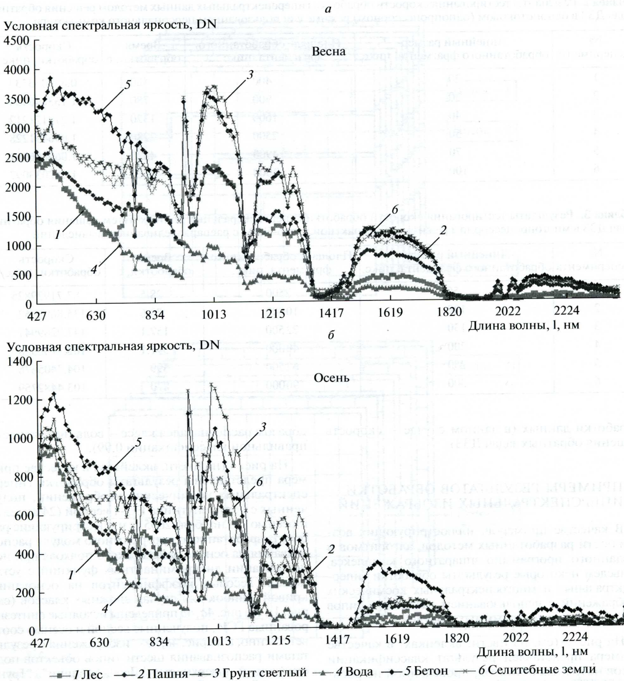
Рис. 5. Спектры различных объектов местности, выделенных в результате классификации гиперспектральных космических изображений, полученных: a – 24 апреля; б – 30 ноября 2005 г. с помощью аппаратуры Nuregion спутника EO-1.
